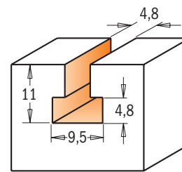
Tekeningen in schaal 1:1 Profils à échelle 1:1
