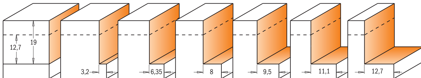
Tekeningen in schaal 1:1 Profils à échelle 1:1
