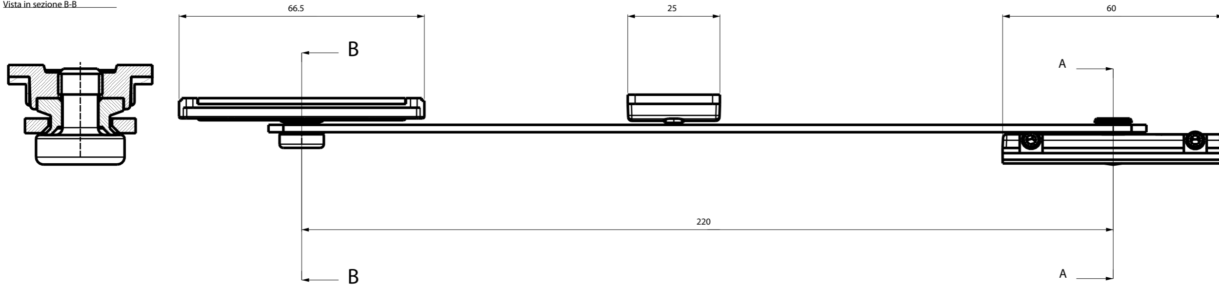
Vista in sezione B-B
