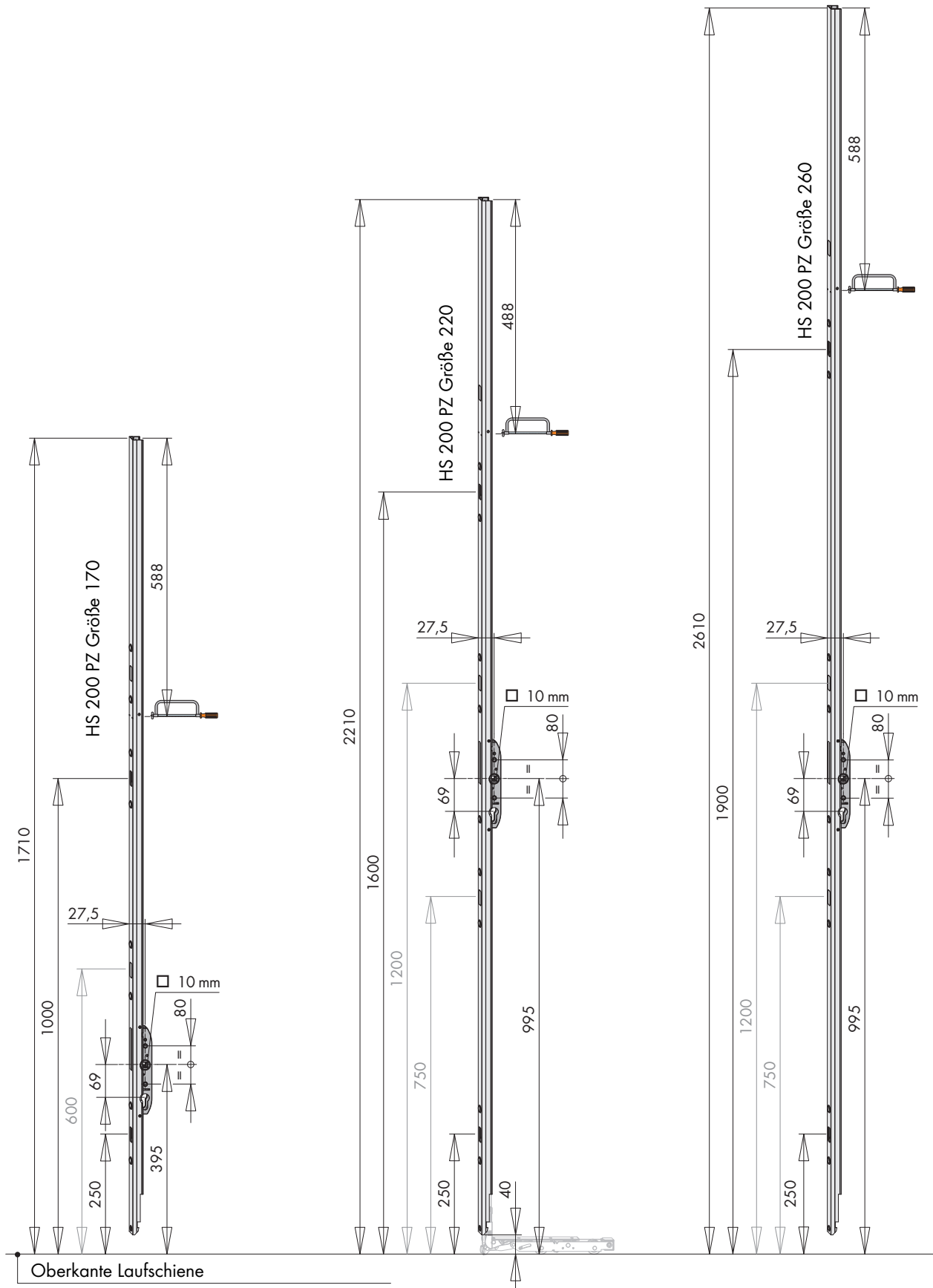
Abb. 187: Getriebe PORTAL HS 200 PZ
