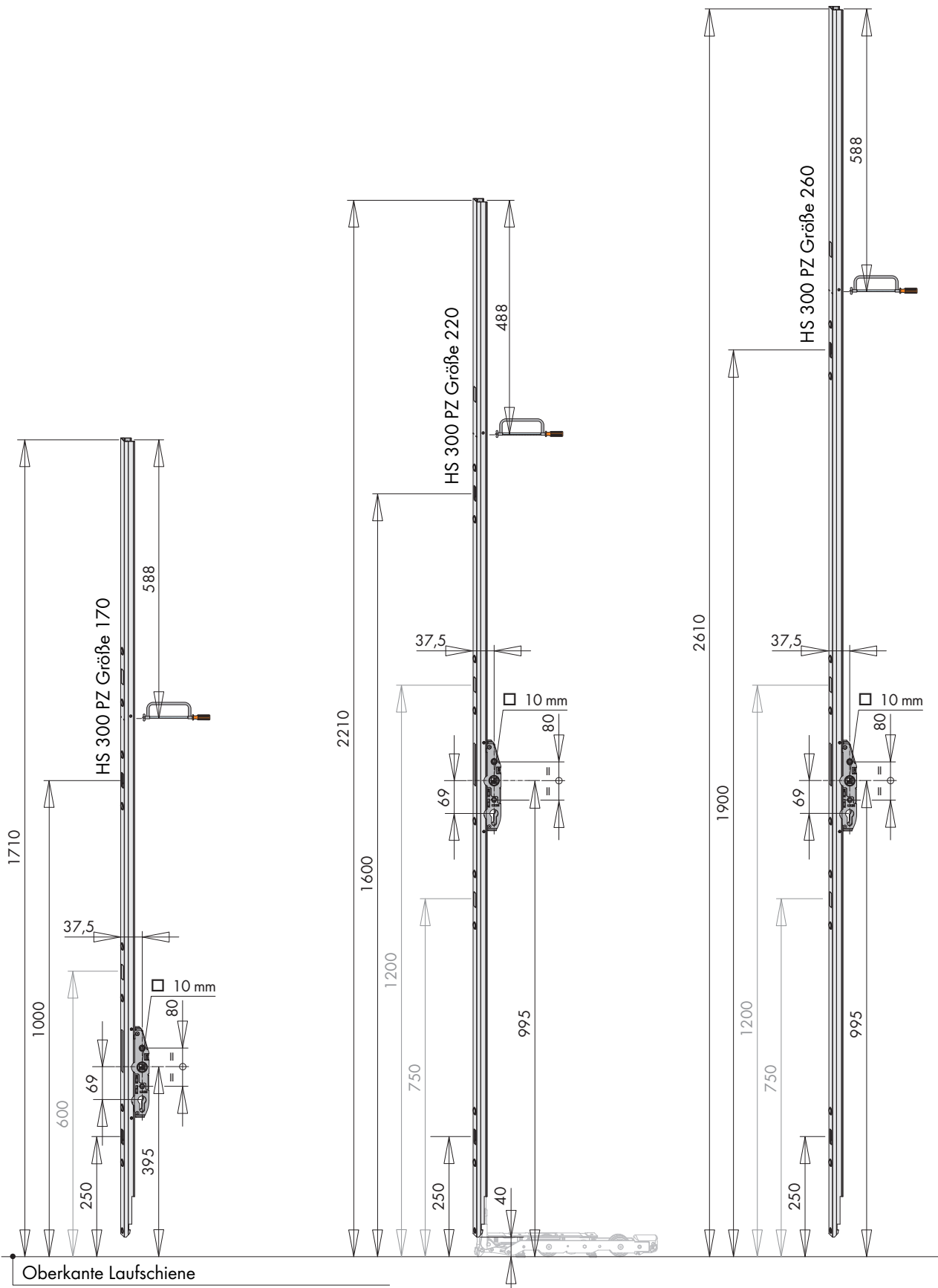
Abb. 190: Getriebe PORTAL HS 300 PZ
