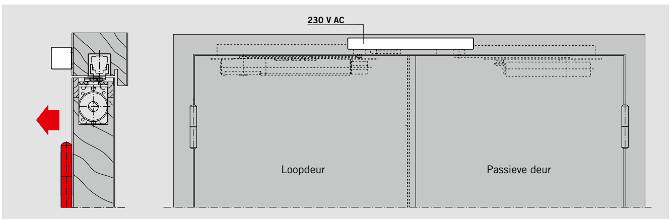
Rookmeldcentrale RMZ aan de scharnierzijde in combinatie met vrijloopdeurdranger ITS 96 FL en G 96 GSR Voorbeeld: DIN-linkse deur, DIN-rechtsse deur spiegelbeeldig
