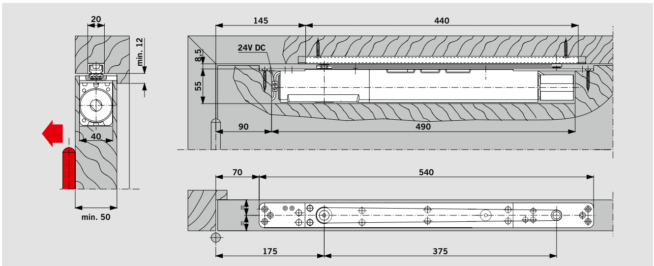
Deurdranger ITS 96 FL met glijarm G 96 N20 in een houten deur
