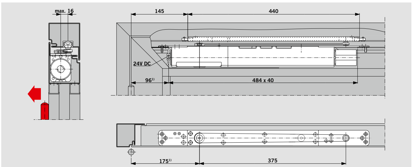
Deurdranger ITS 96 FL met glijarm G 96 N20 in een profiel deur
