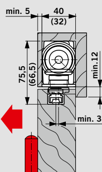
Afbeelding ITS 96 EN 3-6 ( ) Maten = ITS 96 EN 2-4
