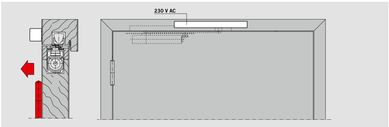
Rookmeldcentrale RMZ aan de scharnierzijde in combinatie met ITS 96 EMF Voorbeeld: DIN-linkse deur, DIN-rechtsse deur spiegelbeeldig
