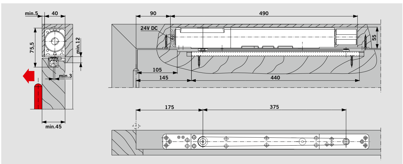
Deurdranger ITS 96 FL met glijarm G 96 N20 in een houten kozijn in kopmontage
