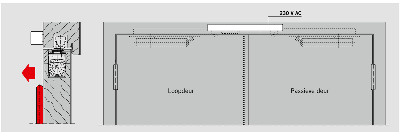
Rookmeldcentrale RMZ aan de scharnierzijde in combinatie met ITS 96 GSR-EMF Voorbeeld: DIN-linkse deur, DIN-rechtsse deur spiegelbeeldig
