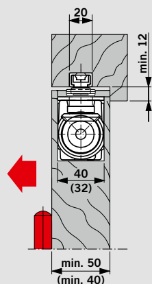
Afbeelding ITS 96 EN 3-6 ( ) Maten = ITS 96 EN 2-4
