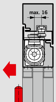
Afbeelding ITS 96 EN 3-6 ( ) Maten = ITS 96 EN 2-4
