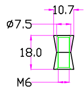
GROMMET
