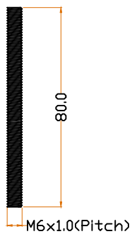
STUD M6x80
