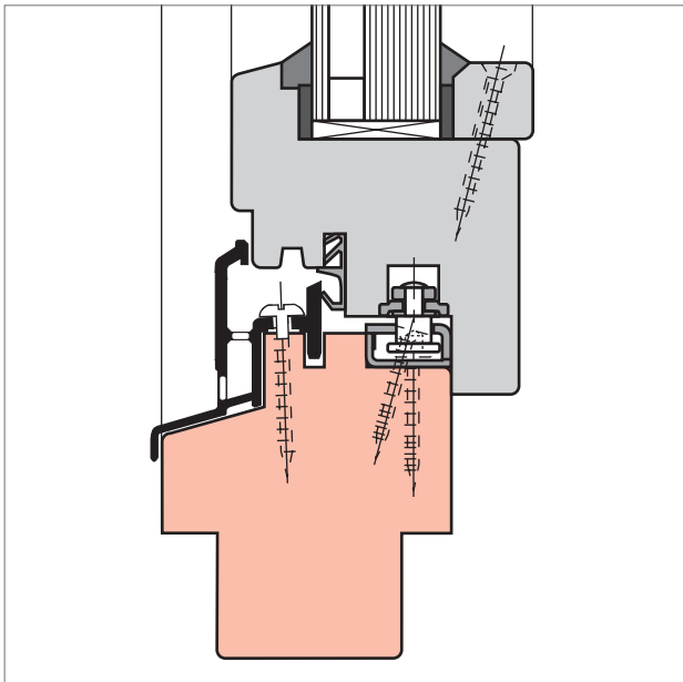
Vertikalschnitt M 1:2
