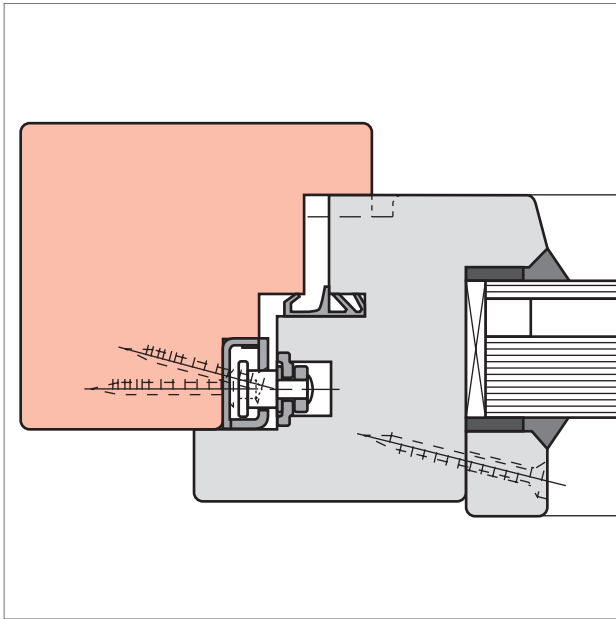
Horizontalschnitt M 1:2
